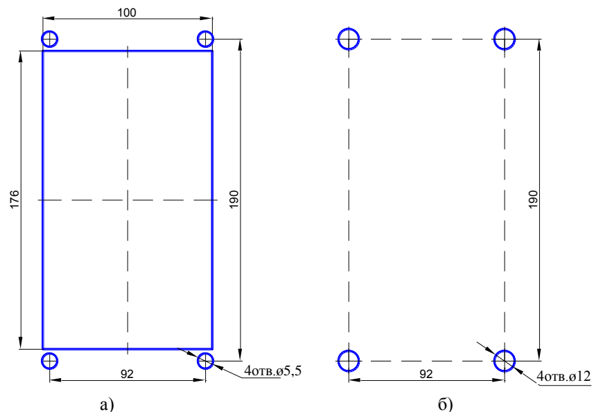
Рис 1. Разметка под крепление DP400-RD24 а) снаружи; б) изнутри.
